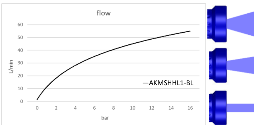
Débit d'eau à la buse complètement ouverte, en fonction de la pression
