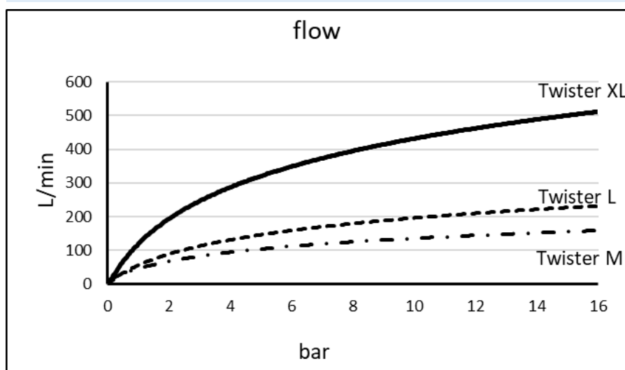
Débit d'eau avec une buse complètement ouverte, en fonction de la pression
